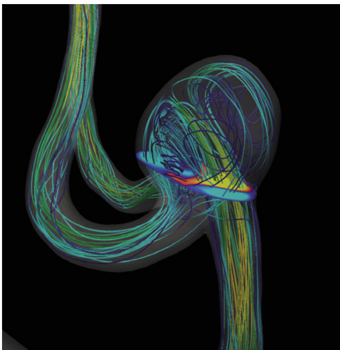
Datasimulering av blodstrøms hastighet og -retning i et aneurisme lokalisert i delingen til en hjernearterie. Simulering og visualisering er utført av Simula Research Laboratory, Oslo.
